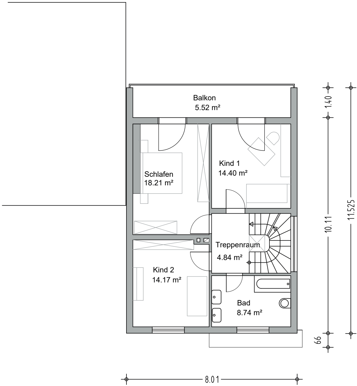
GRUNDRISS OBERGESCHOSS
