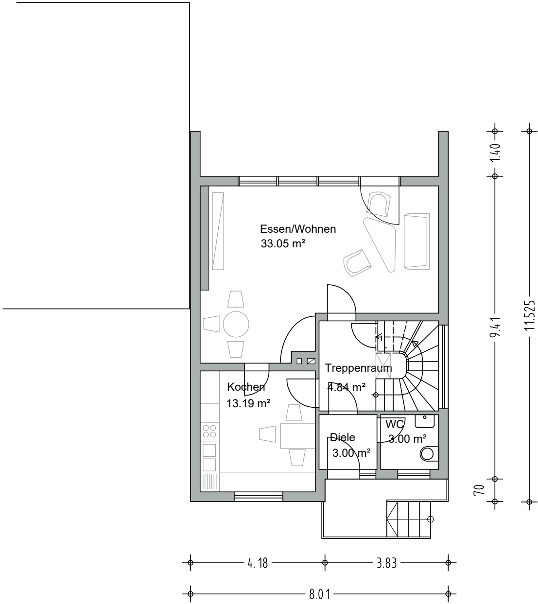
GRUNDRISS ERDGESCHOSS
